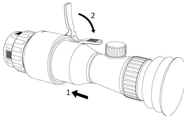
Figura 2-3 Instalar la mira telescópica diurna
