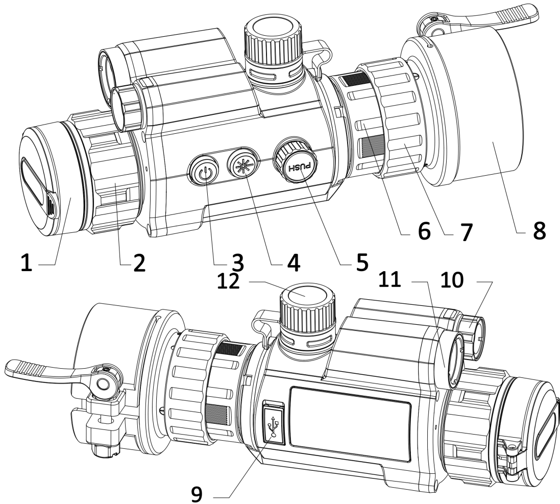
Figura 1-1 Aspecto del dispositivo
