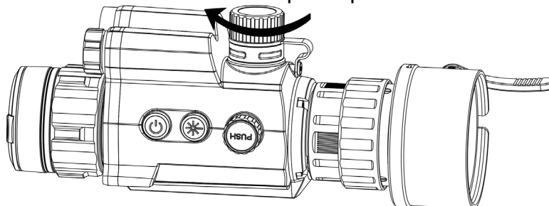
Figura 2-6 Cerrar la tapa de la batería
