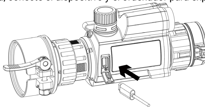
Figura 2-1 Conexión del cable
