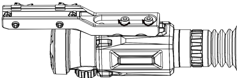
Figura 2-6 Asegurar el dispositivo
