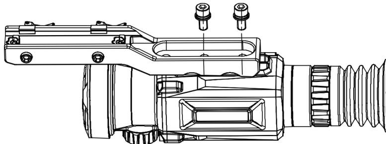
Figura 2-5 Insertar los tornillos
